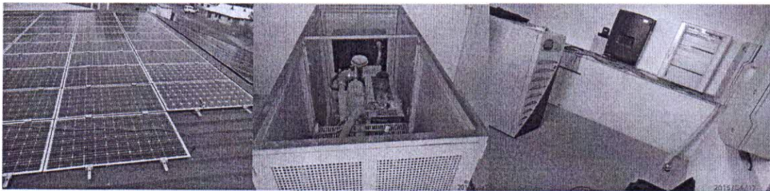
Tetto con pannelli solari. Generatore 3 fasi 25 Kva. Sala controllo sistema fotovoltaico per l'Ospedale Statale di Rumbek.
